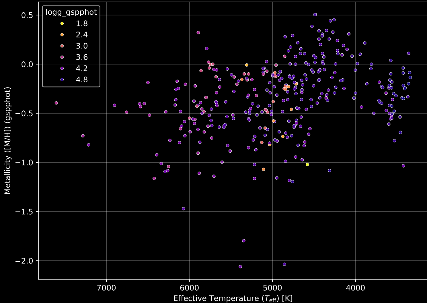
APOGEE DR17 Field: [ORPHAN-4] Stellar Population Parameters (n= 345)
